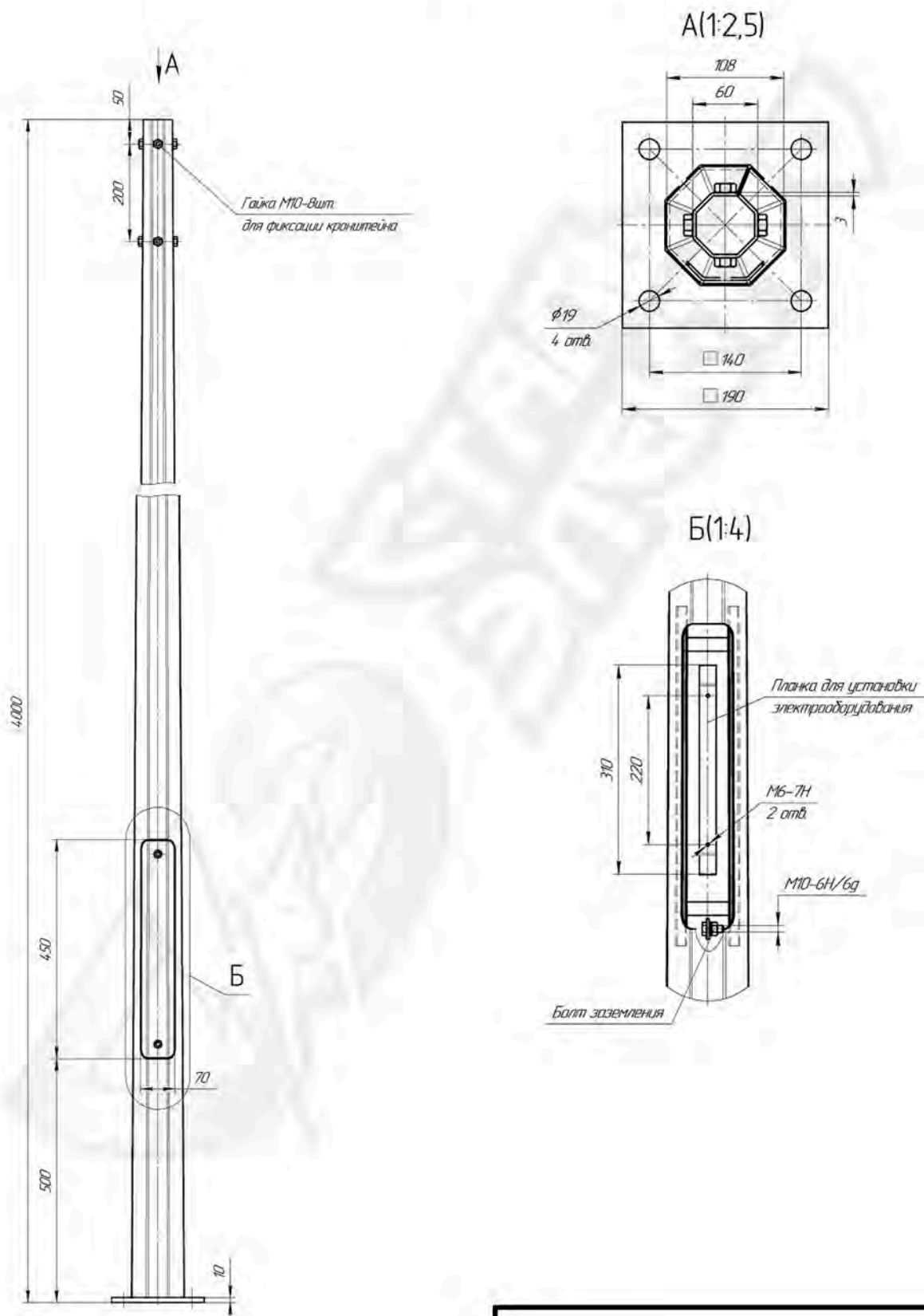
Рис. 1 Основные габаритные и присоединительные размеры
